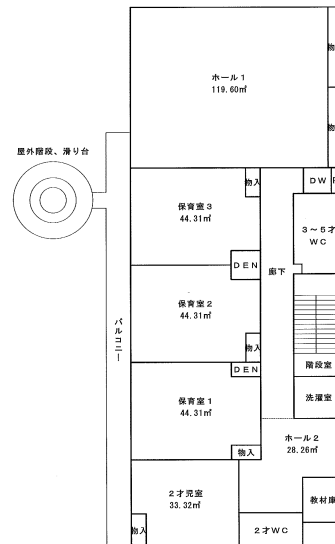
2階平面図
