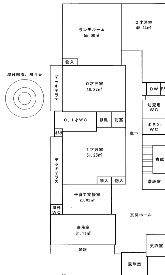
1階平面図
