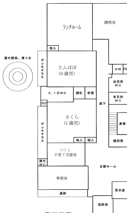
1 階平面図
